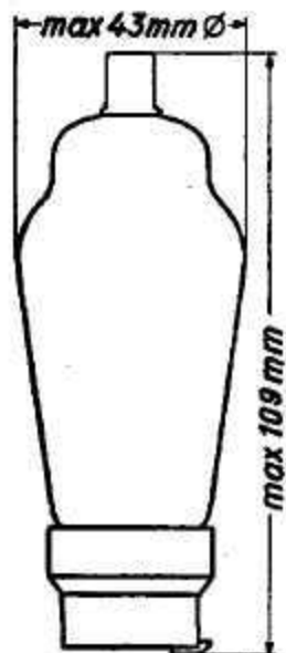
Kolbengröße
